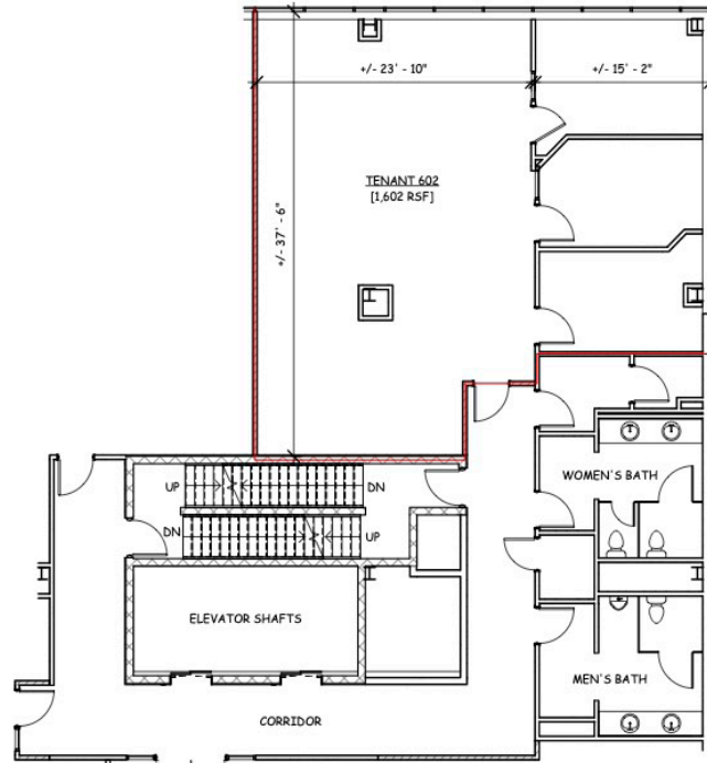
① TENANT 602 & CORE 1/8" = 1'-0"
